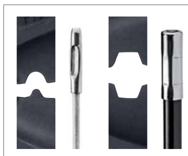
Perfiles de prensado
