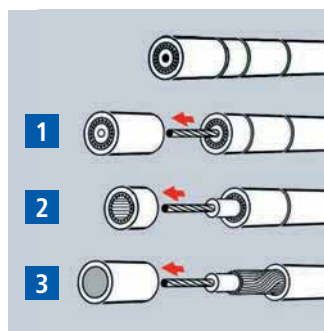
Pelado de cables coaxiales en 3 pasos
